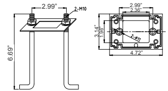
BOL-505-ABK 6.69"(H) x 2.99"(W)
