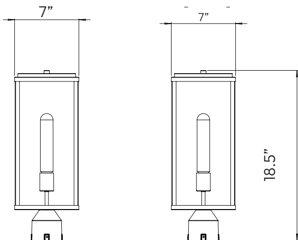
Technical Drawing: 7" (D) x 7" (W) x 18.5" (H)
