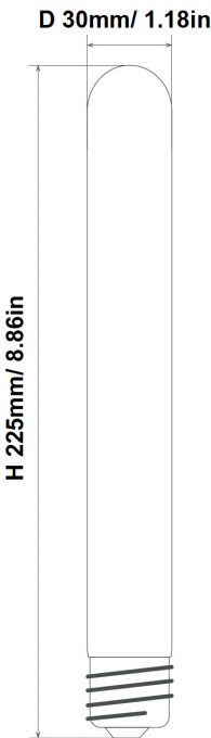
8.8"(H) x 1.18"(W)
