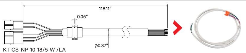
KT-CS-NP-10-18/5-W /LA
