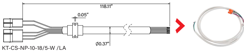
KT-CS-NP-10-18/5-W /LA
