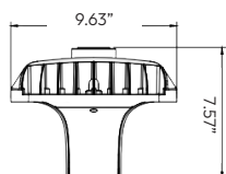
Technical Drawing: 9.63" (D) x 26.25" (W) x 7.57" (H)
