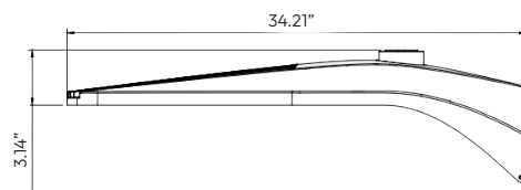
Technical Drawing: 12.82" (D) x 34.21" (W) x 8.13" (H)
