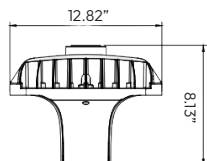
Technical Drawing: 12.82" (D) x 34.21" (W) x 8.13" (H)
