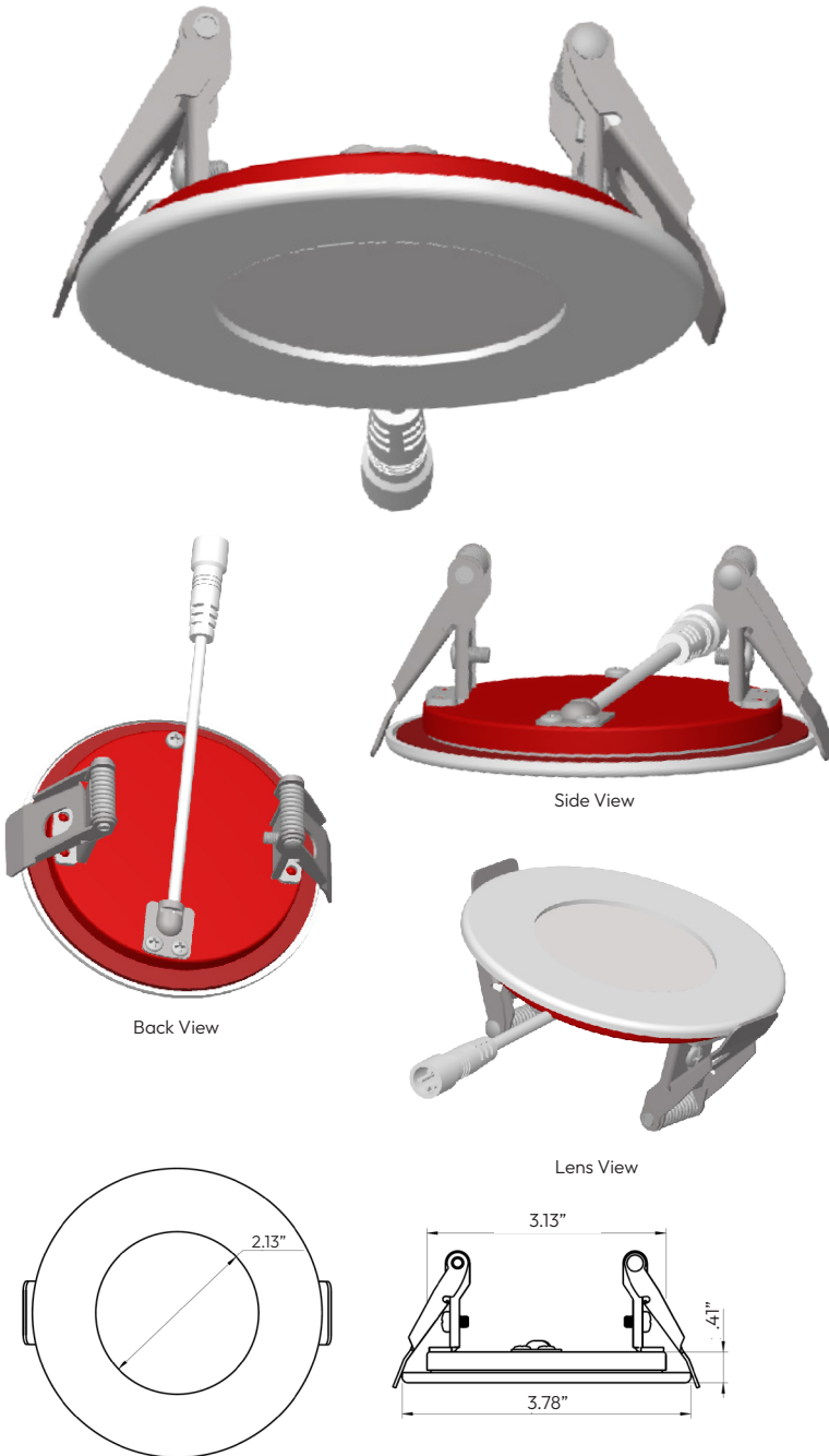
Technical Drawing: 3.78" (D) x 3.13" (W) x .41" (H)
